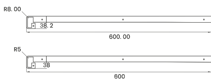
Listwa łączeniowo-szczelinowa
